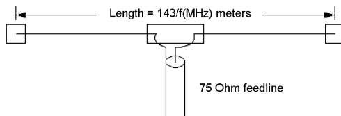
Figura 15 – Diagrama de antena dipolo (figura obtida no Wikipédia)
