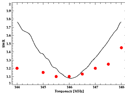
Figura 14 - Gráfico de variação da estacionária numa antena para faixa de 2m. Os pontos vermelhos indicam os valores medidos e a curva marca a estacionária teórica máxima.
