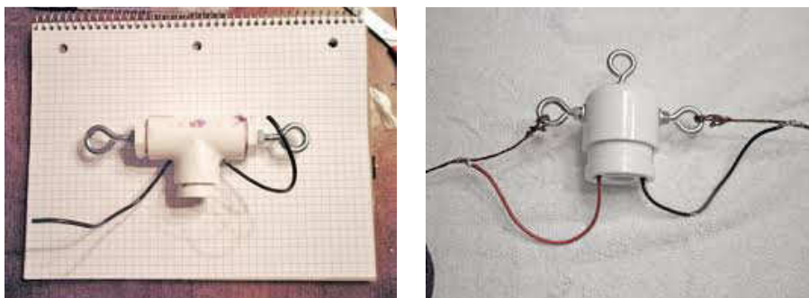
Figura 16 - fotos de K4ICY – isolador central para dipolo
