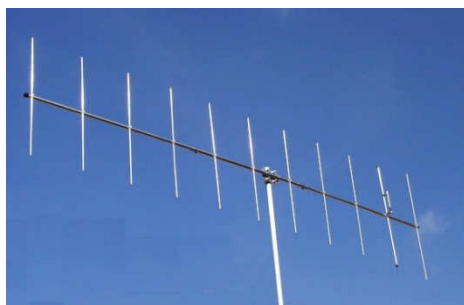
Figura 20 - yagi com 11 elementos para 2m. Como cada dipolo é pequeno (50 cm cada lado) nessa faixa é possível usar antenas com muitos parasitas. Nove diretores e um refletor
