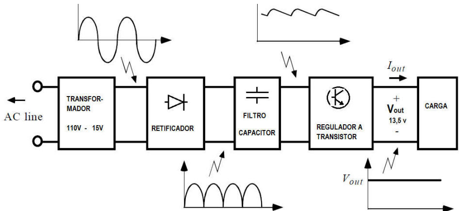
Figura 28 - Diagrama em blocos da fonte de alimentação
